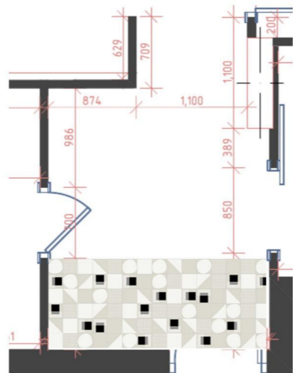
План сверху
